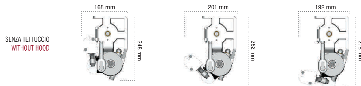
INGOMBRI / BULKS INCLINAZIONE / INCLINATION 5° INCLINAZIONE / INCLINATION 40° INCLINAZIONE / INCLINATION 70°
