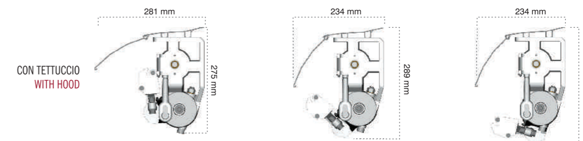
INGOMBRI / BULKS INCLINAZIONE / INCLINATION 5° INCLINAZIONE / INCLINATION 40° INCLINAZIONE / INCLINATION 70°
